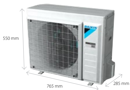
Unidade exterior ERLA03DV Classe 3,5 kW
