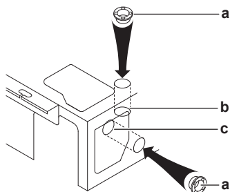
a Casquilho de resina (acessório) b Pré-orifício (para entrar a partir do topo)
