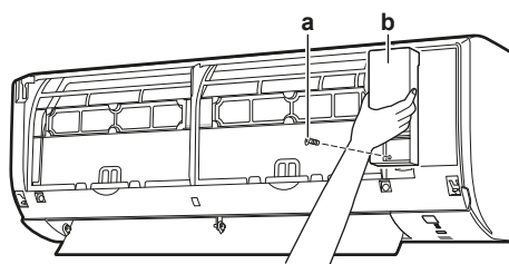
a Parafuso da tampa de serviço b Tampa para assistência técnica
