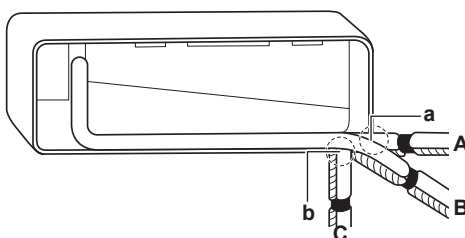
A Tubagem no lado esquerdo B Tubagem na parte traseira esquerda C Tubagem na parte inferior esquerda a Retire a tampa do orifício do tubo aqui para a tubagem no lado esquerdo b Retire a tampa do orifício do tubo aqui para a tubagem na parte inferior esquerda
