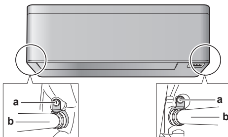
a Parafuso de fixação do isolamento b Mangueira de drenagem
