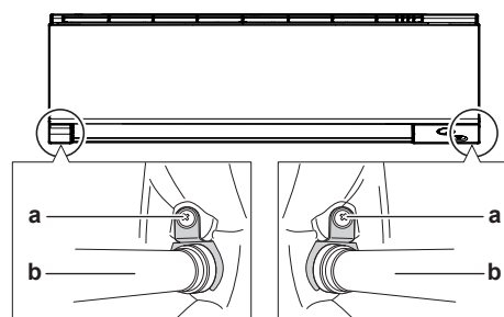
a Parafuso de fixação do isolamento b Mangueira de drenagem
