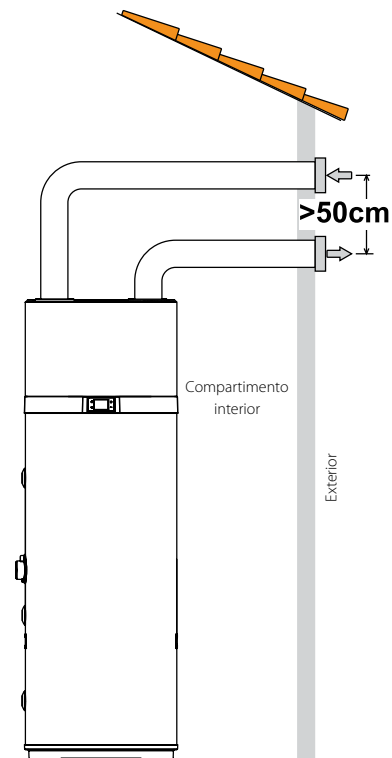
Fig. 2 - Exemplo de ligação da descarga de ar
