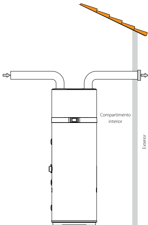
Fig. 1 - Exemplo de ligação da descarga de ar
