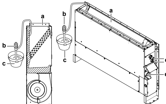
a Saída de ar b Bomba portátil c Balde d Tubos de arrefecimento e Saída de drenagem
