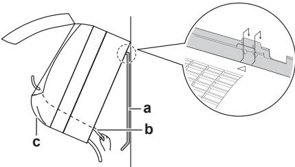
a Placa de montagem (acessório) b Cabo de interligação c Guia dos fios
