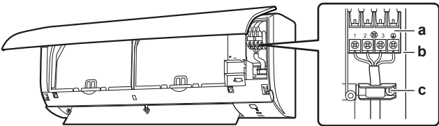
a Placa de bornes b Placa de componentes eléctricos c Braçadeira de cabos
