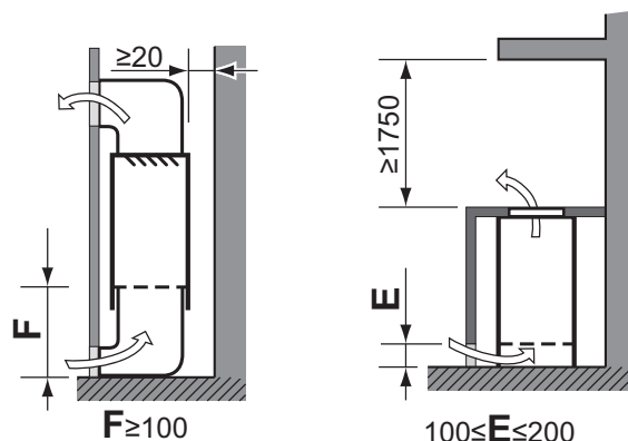
Tipo de montagem na parede
