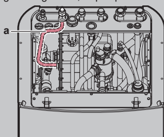
a Tubo de gás refrigerante
